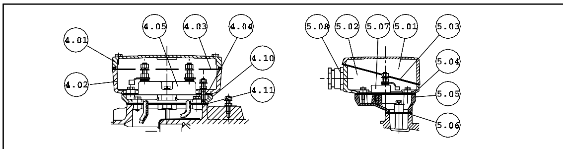
Anschlußsystem für / connection system for Kabelschuhanschluß / connection with cable eye / nur für Type 315 MX, MY, LX, LY / only for type 315 MX, MY, LX, LY /
